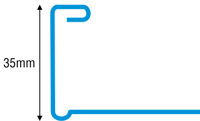
TDF Flange
